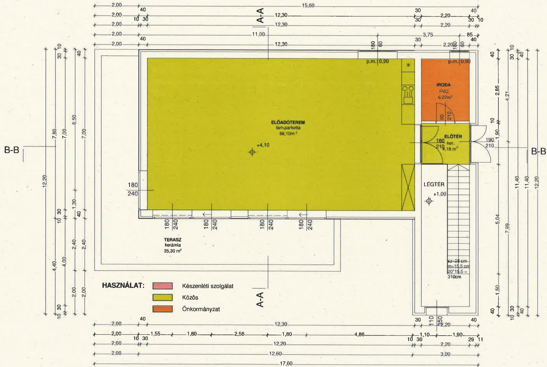
EMELETI ALAPRAJZ M 1:100
